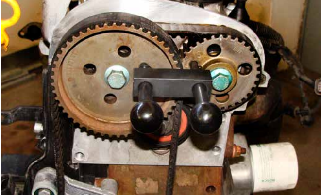
ZAHNRIEMENWERKZEUG 21017
