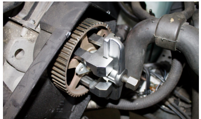
ABZIEHER NOCKENWELLENRAD
