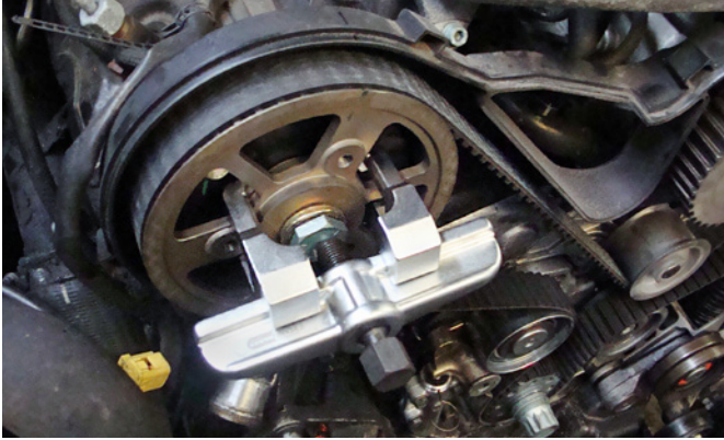
ABZIEHER NOCKENWELLENRAD
