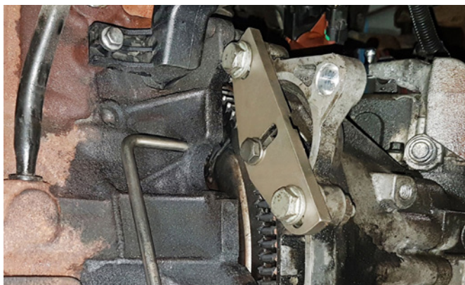
EINSTELLWERKZEUG 103626 / BLOCKIERWERKZEUG 50017
