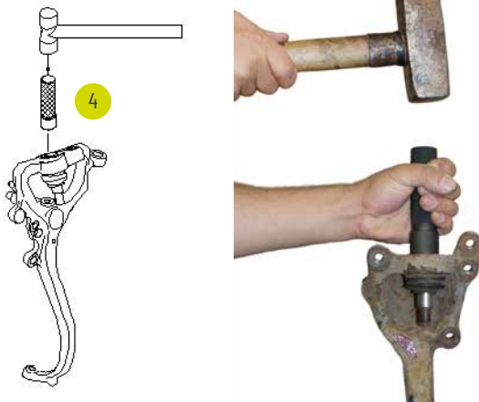
AUSBAU DES ALTEN KUGELGELENKS BEI W220
