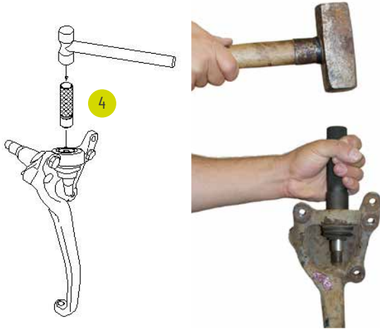
AUSBAU DES ALTEN KUGELGELENKS BEI W123, W126
