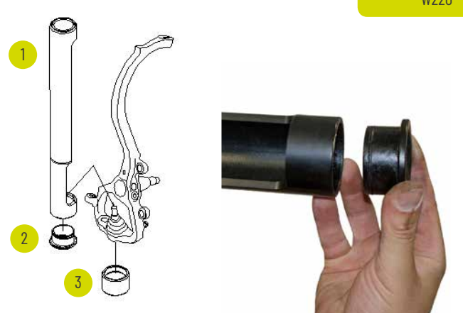
EINPRESSEN DES KUGELGELENKS BEI W220
