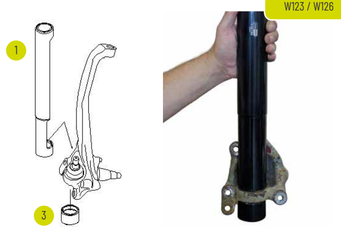
EINPRESSEN DES KUGELGELENKS BEI W123, W126
