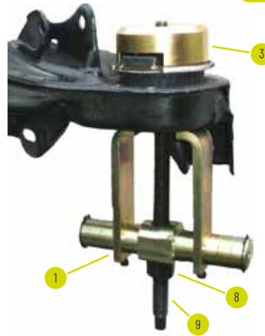
EINBAU VORDERE HINTERACHSLAGER
