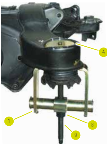
AUSBAU HINTERE HINTERACHSLAGER
